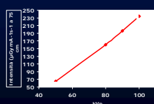
Dipendenza dell'intensità del fascio dai kVp
